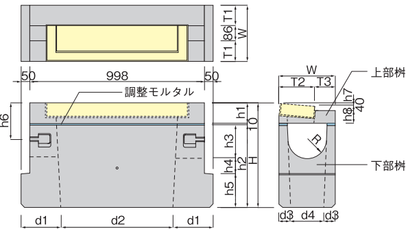
NS-01 φ200～350用
