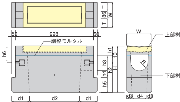
NS-02 \phi 200~250用
