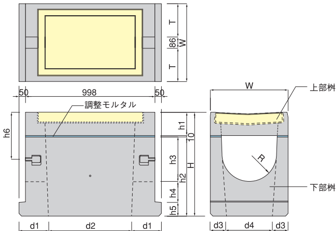
NS-02 \phi 300~600用
