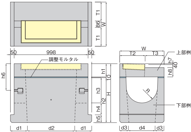
NS-01 φ400～600用
