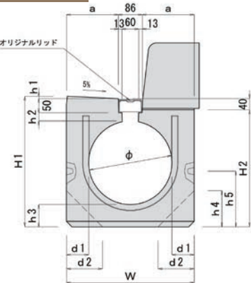
NS-01
