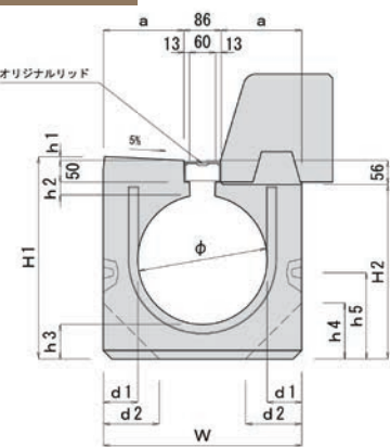
NS-01 H
